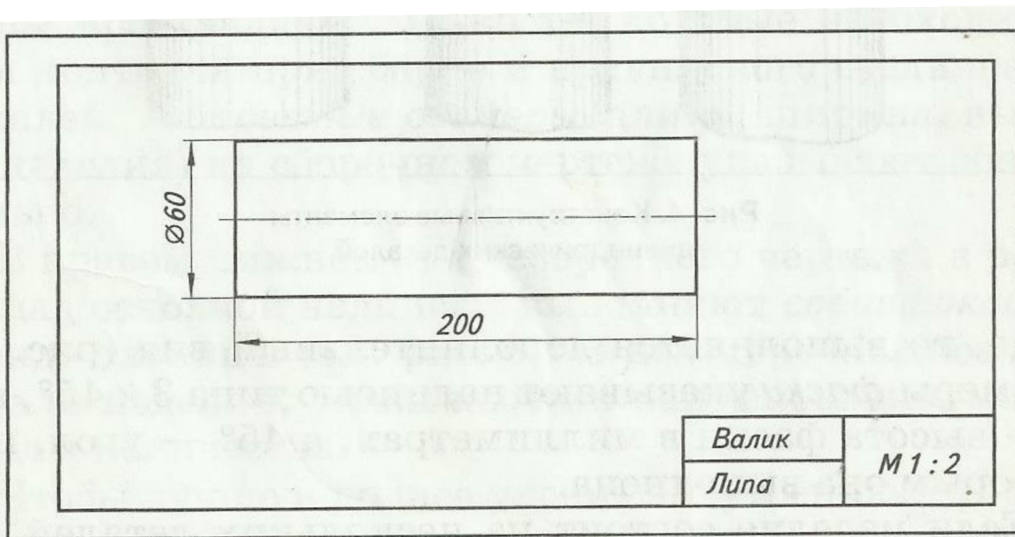
Рис. 2. Чертёж детали цилиндрической формы
